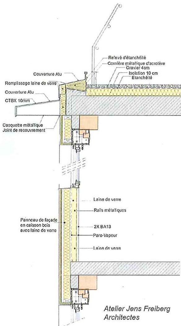
Coupe façade, acrotère, toiture-terrasse
